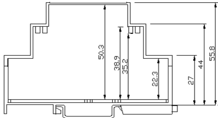
BARRA DIN
