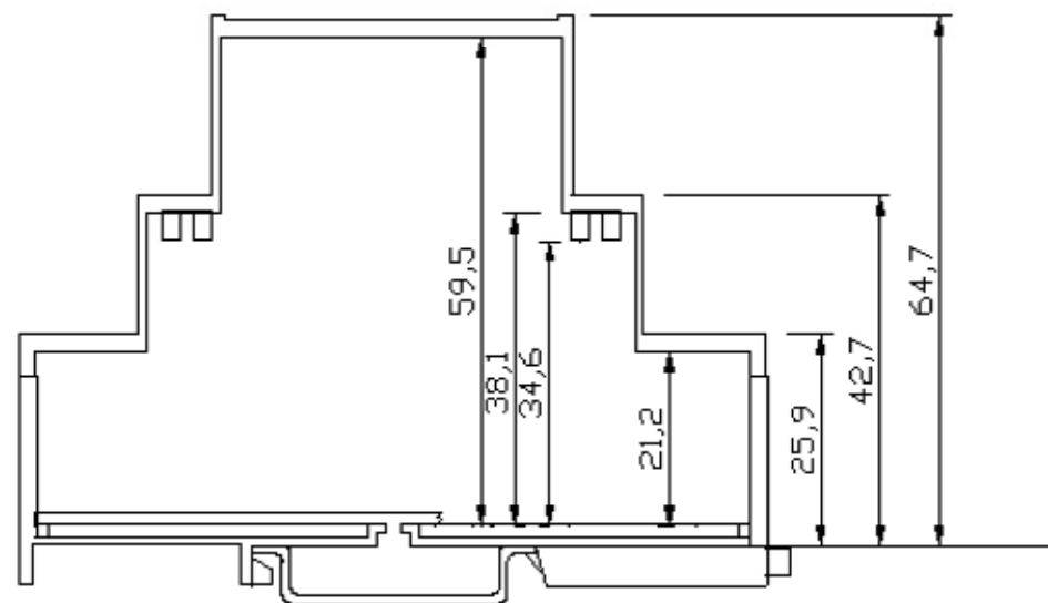
BARRA DIN
